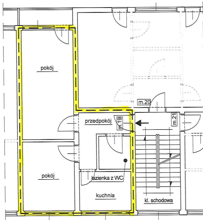
Rzut I-go piętra - fragment skala: n/a
